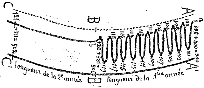
Fig. 4. — Ondulations serpentines ou retraitis stryphnoïdes qui sont des contractions de souffrance.
