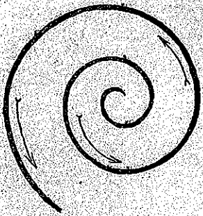
Fig. 1. — Forme théorique d'un tourbillon de destinées.
